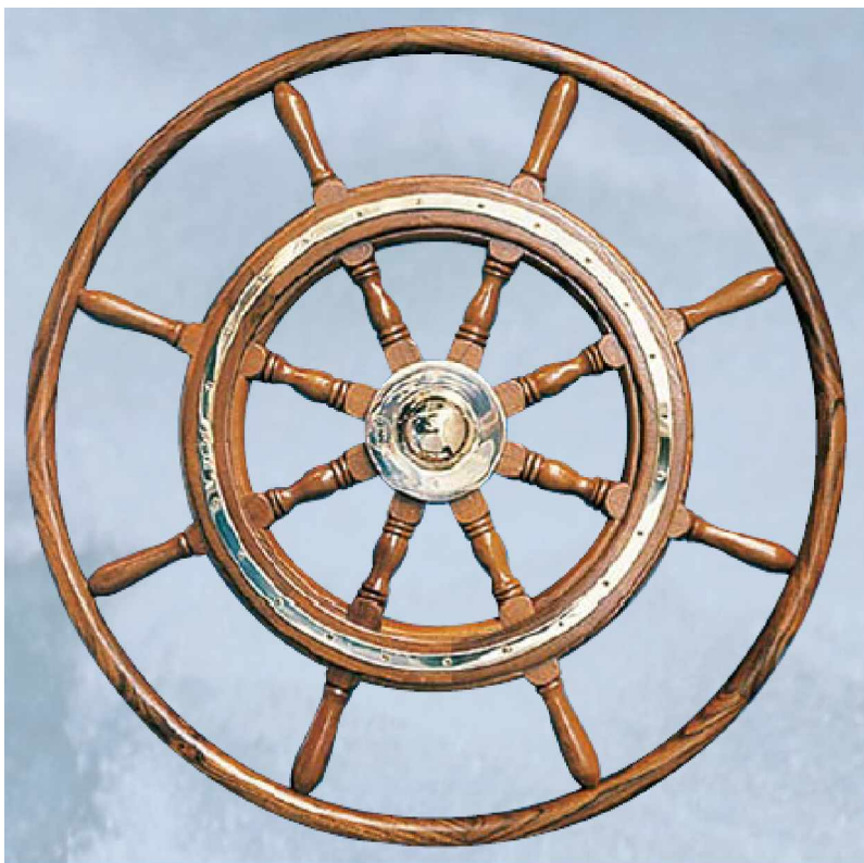
07. Штурвал с восемью спицами, тиковым ободом и латунным или хромированным фитингом
